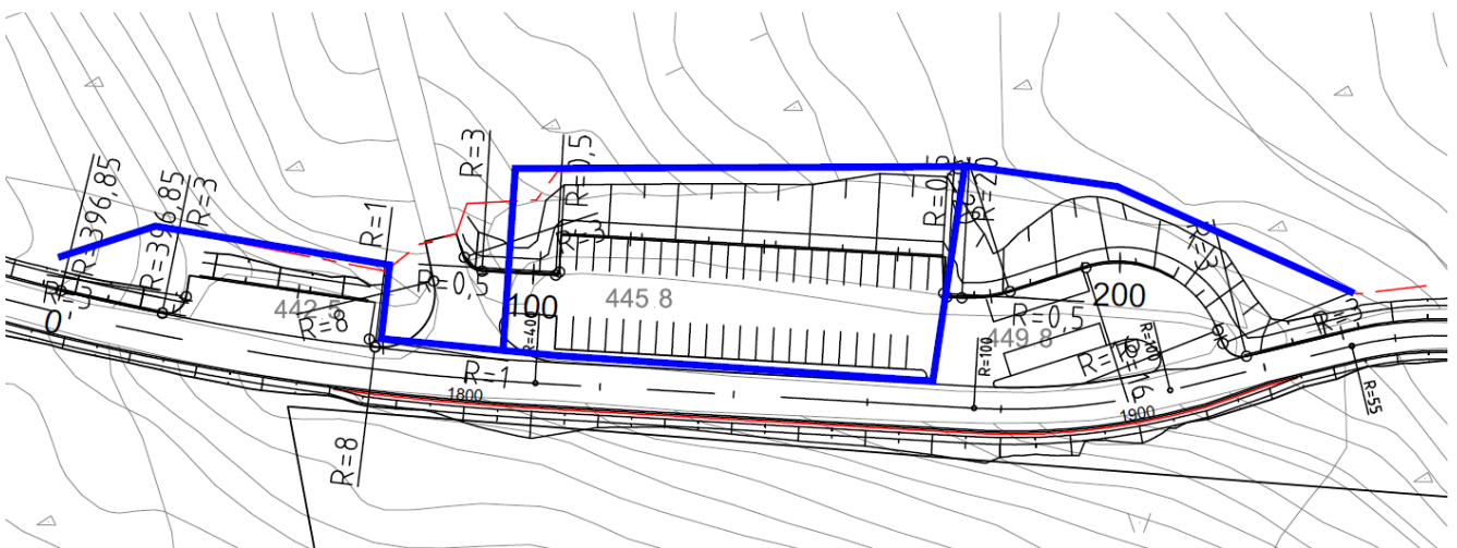
Kuva 14. Tunturitien valitun vaihtoehdon pysäköintialueen asemapiirros.
