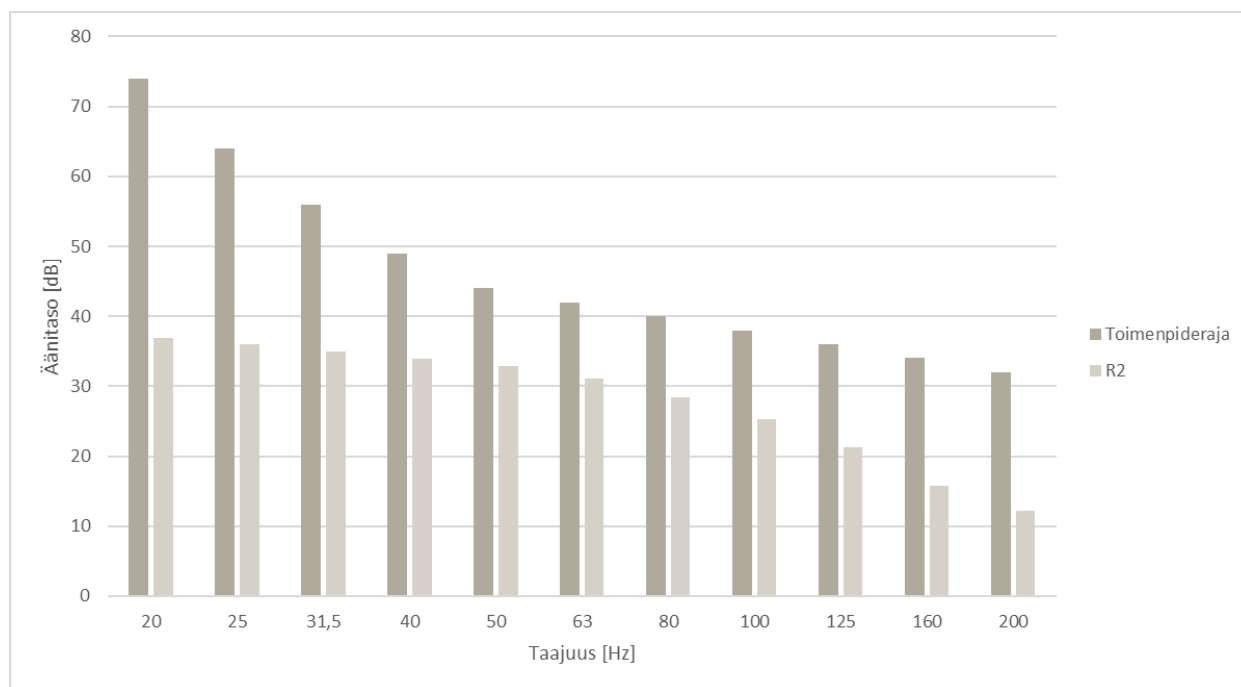
Kuva 5: Matalataajuisen sisämelun tasot reseptorin R2 kohdalla.
