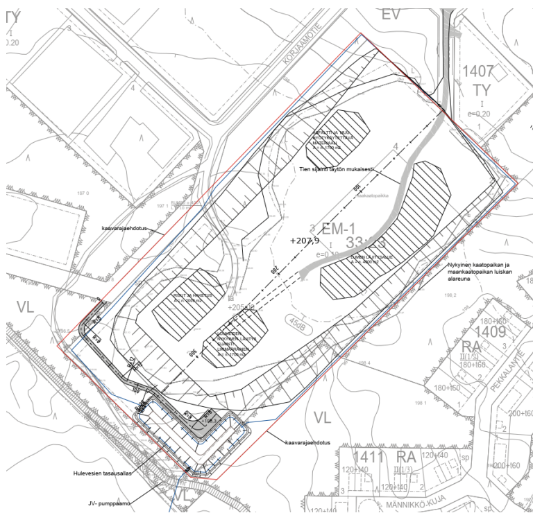
Ote nykyisen maanjäätysalueen täyttösuunnitelman asemapiirustuksesta (FCG, 1.4.2020).
