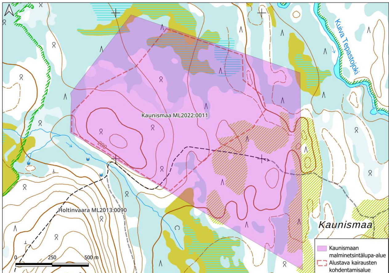
Kuva 1. Kaunismaan malminetsintäalue ja sen alueella suunniteltujen kairausten alustava kohdealue.
